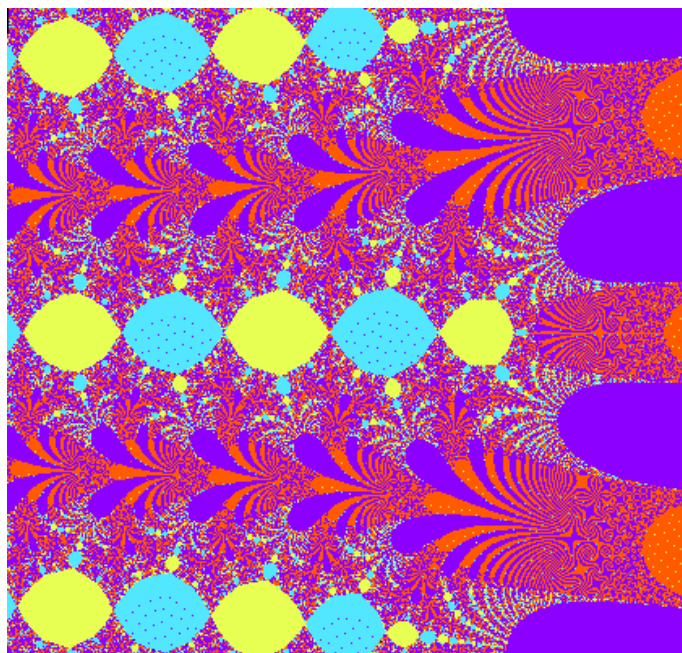
図 1: f(z) = \lambda ze^z のファトウ集合
