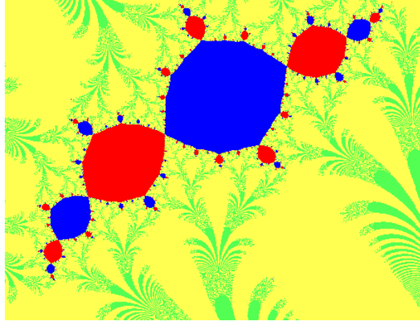
図 2: \lambda = 0.0577688 - 0.0721882i a = 4 - 2.8i
